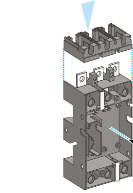
Mühürlenilebilir terminal koruyucuları
