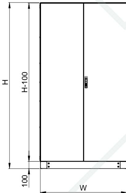
ÖN GÖRÜŞÜ
