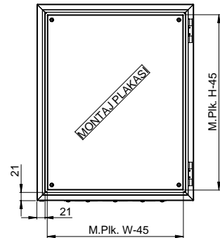
İÇ GÖRÜNÜŞ
