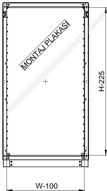
İÇ GÖRÜŞÜ
