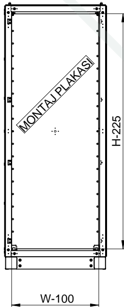
İÇ GÖRÜNÜŞ
