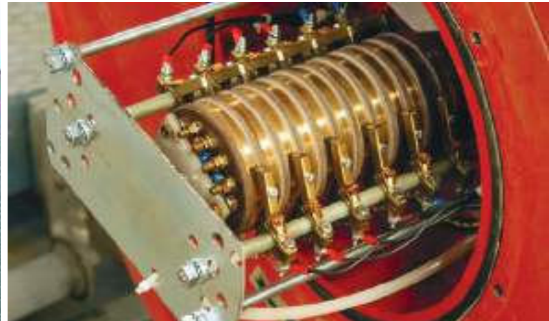
Endüstride Teknik Çözümler TAMBUR ENERJİ AKTARIM KOLLEKTÖRÜ (10A./40A. 3/16 kutuplu çeşitlerimizde.)
