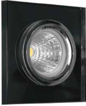
MOL559 3.00$ | SİYAH KASA | ALÜMİNYUM GÖVDE | AMPÜL HARIÇ | KOLİ 100 ADET | IP20
