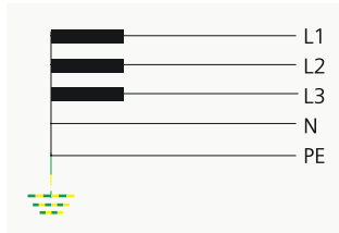
TN-S Sistem
