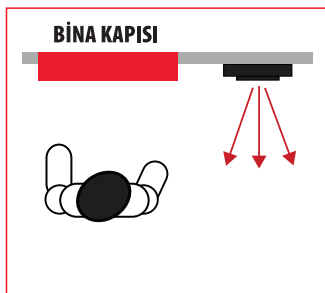
YANLIř MONTAJ
