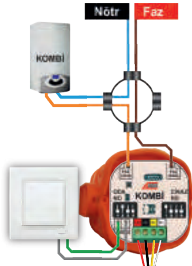
KOMBİ BAĞLANTISI
